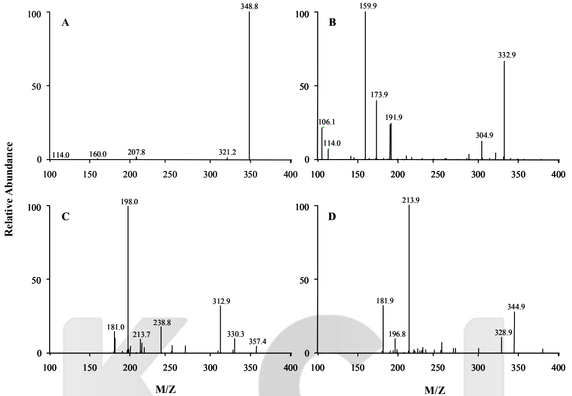
Fig. 6. ESI tandem mass spectra of standard \beta lactams; (A) Amoxicillin (B) Ampicillin (C) Pencillin G (D) Penicillin V.
