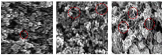
Fig. 3. SEM images of TiO 2 -MWNT (0.1, 0.25, 0.5 wt%).
