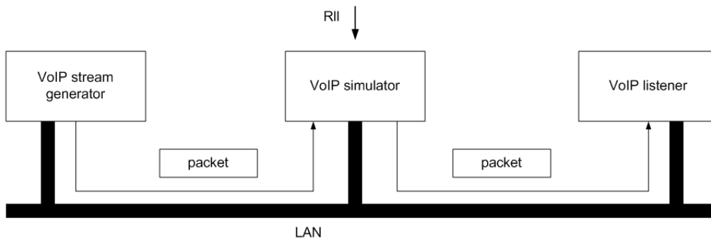
Fig. 5. VoIP testbed
