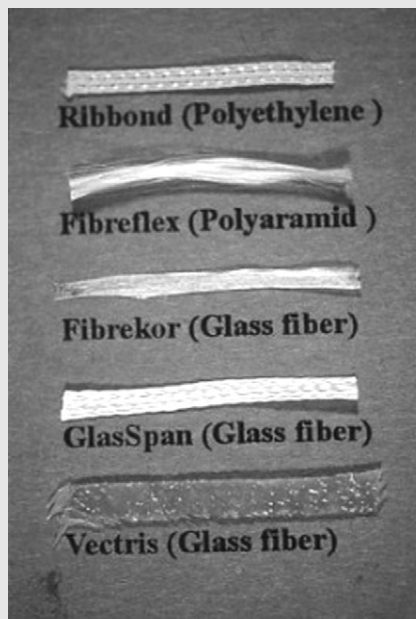
그림 2 섬유강화 복합재료에 사용되는 여러 가지 섬유들. 위로부터 reno-woven 짜임의 폴리에틸렌 섬유(Ribbond®), 폴리아로마틱 폴리아마이드 섬유(Fibreflex®), 미리 레진 기질에 적셔진 유리 섬유 (Fibrekor®), 뿔 형태의 유리섬유 (GlasSpan®), 미리 레진 기질에 적셔져 있고, bi-directional한 배열의 유리 섬유(Vectris Frame®).
