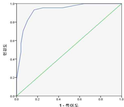
그림 2. ROC 곡선
