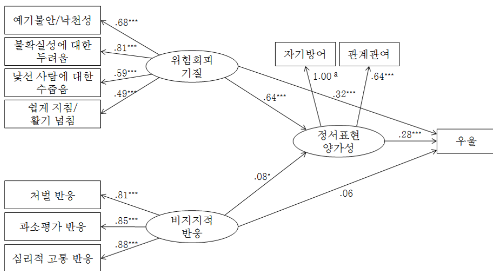
그림 2. 구조방정식 모형(최종모형)
