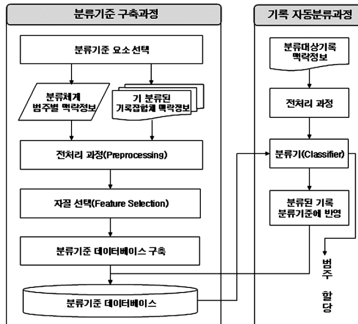
<그림 1> 기록 자동분류시스템 구성도
