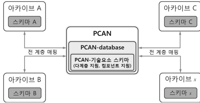
〈그림 4〉 통합 스키마형 PCAN(DA형)
