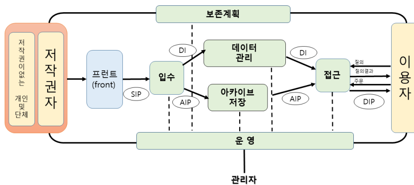
<그림 7> 민중가요 기록물에 적합한 OAIS 참조모형
