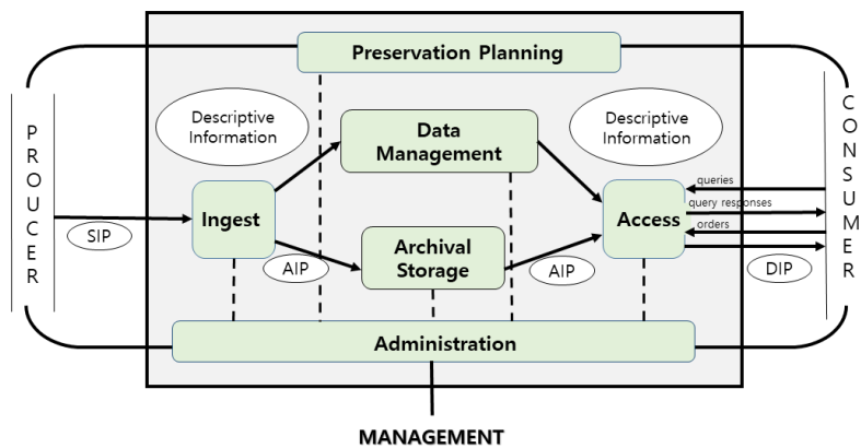
〈그림 6〉 OAIS 기능 간의 연관 관계
