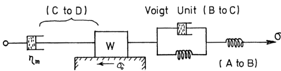
Fig. 3 Bingham-Voigt Model
