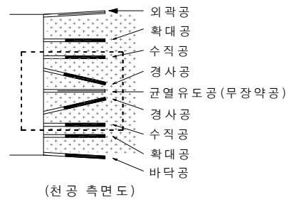
(천공 측면도)
