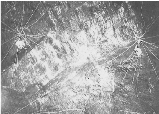
그림 3. COPA-w Cut 발파공법의 천공 배열
