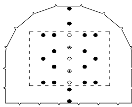
(천공 배열도)
