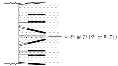
(천공 측면도)
