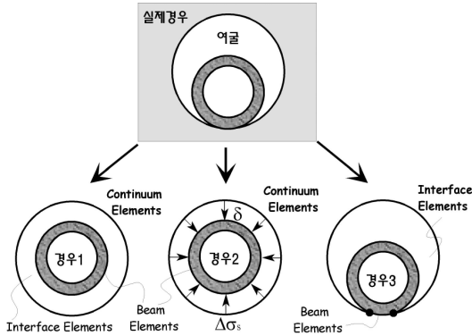
그림 10. 여굴에 대한 모델링
