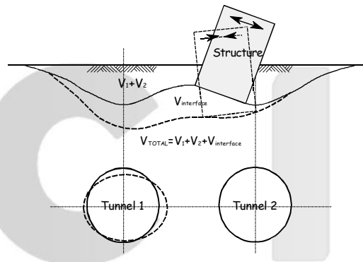
그림 12. 근접터널에 있어서 중첩방법에 의한 지표침하
