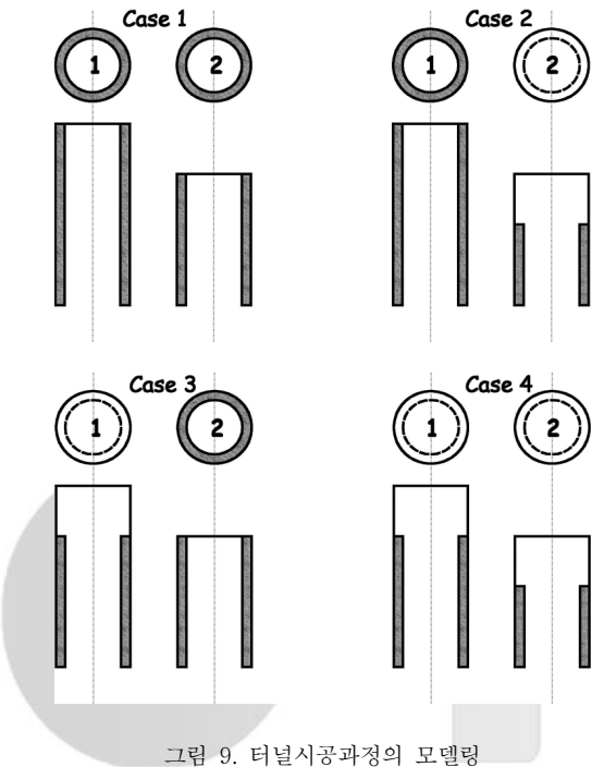
그림 9. 터널시공과정의 모델링
