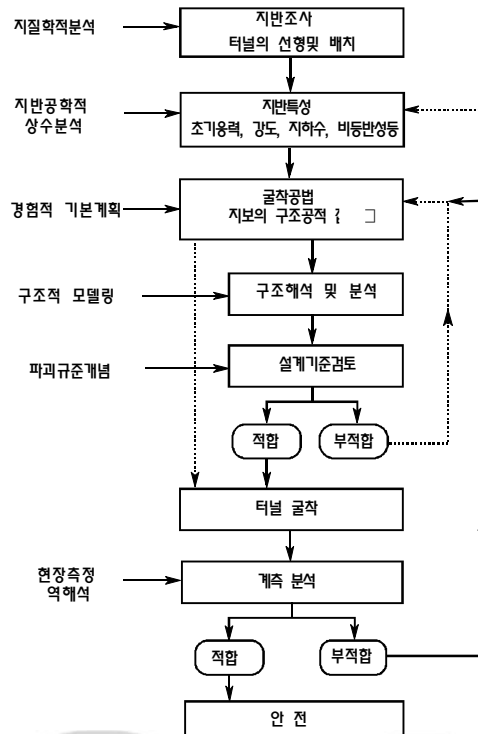
그림 1. 터널의 설계과정 흐름도
