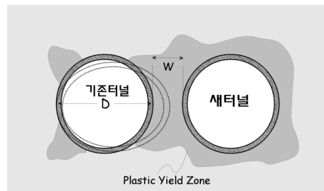
그림 4. 두 평행터널사이의 상호 거동
