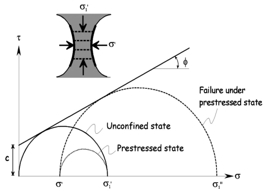
그림 7. 지반의 응력상태 (Prestress 전후)
