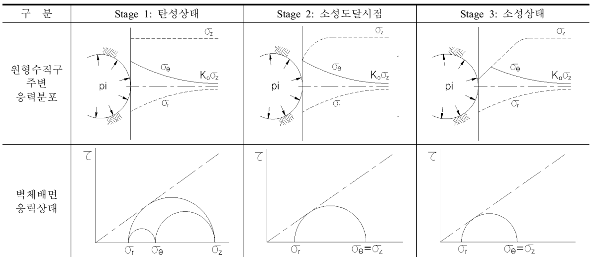
그림 4. 원형수직구 배면지반의 응력분포 (Wong & Kaiser, 1988a)
