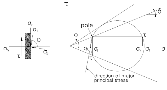
그림 18. 배면지반 응력상태에 대한 Mohr원 (Paik & Salgado, 2003)
