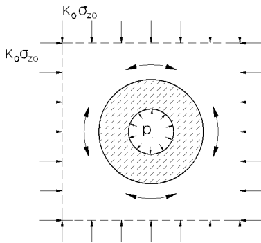
(a) 수평면에서의 아칭
