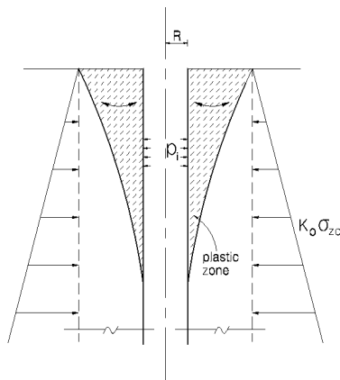
(b) 연직면에서의 아칭
