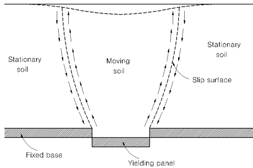
그림 1. 아칭효과에 의한 응력 재분배 (Terzaghi, 1943a)
