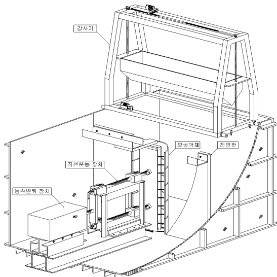
그림 12. 모형벽체 형태
