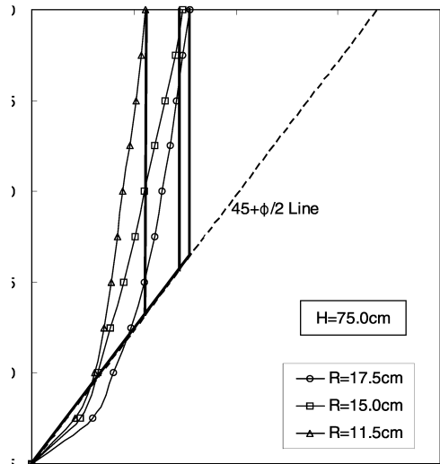
그림 15. 파괴면 형상에 대한 벽체반경의 영향
