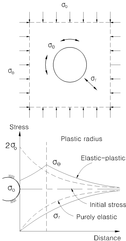
그림 2. 원형공동에 의한 아칭효과 (Fara & Wright, 1963)
