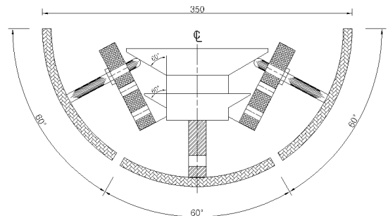
그림 13. 모형벽체 단면
