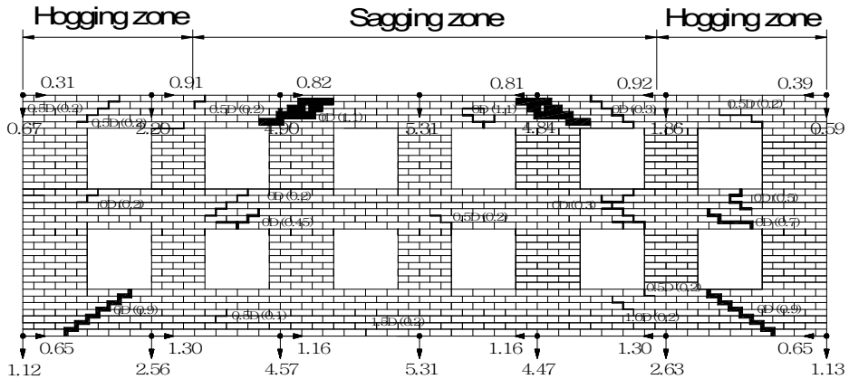
(a) 구조물 변형 및 균열 형상
