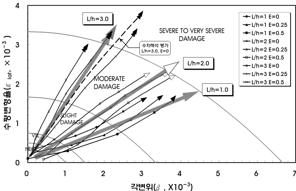
그림 7. 각변위와 수평변형율에 의한 구조물 손상평가
