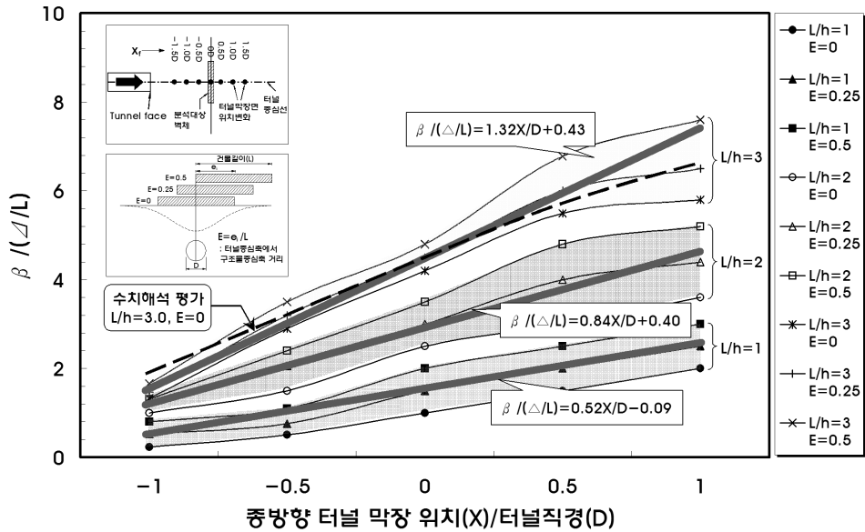
그림 4. 터널굴착시 형상비와 편심거리에 따른 \beta / (\Delta/L) 의 변화
