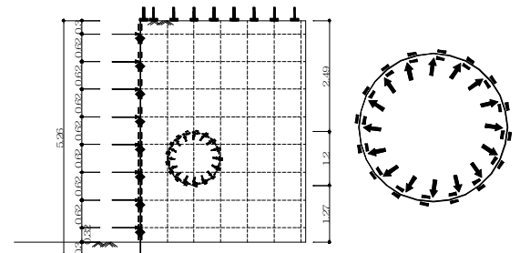
그림 3. 계측기 설치 단면도
