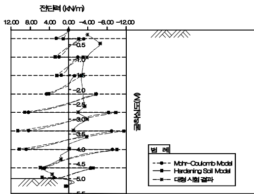
그림 10. 흙막이벽체 전단력도 (선행하중을 가했을 때)
