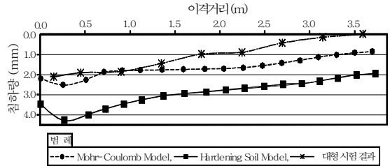
그림 17. 흙막이벽체 배면의 지표침하 (선행하중을 가하지 않았을 때)
