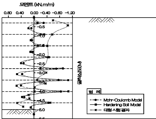
그림 8. 흙막이벽체 모멘트도 (선행하중을 가했을 때)
