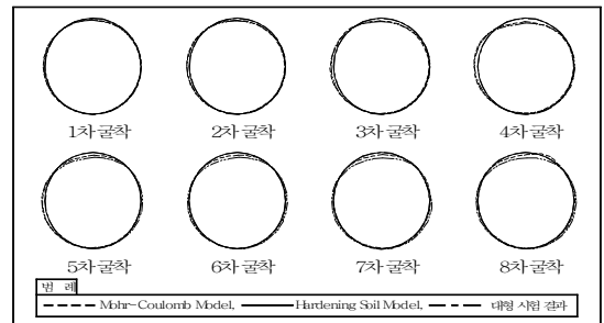
그림 12. 터널 라이닝 내공변위 (선행하중을 가했을 때)
