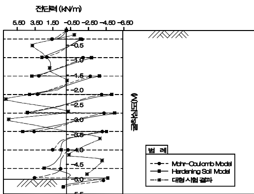
그림 9. 흙막이벽체 전단력도 (선행하중을 가하지 않았을 때)
