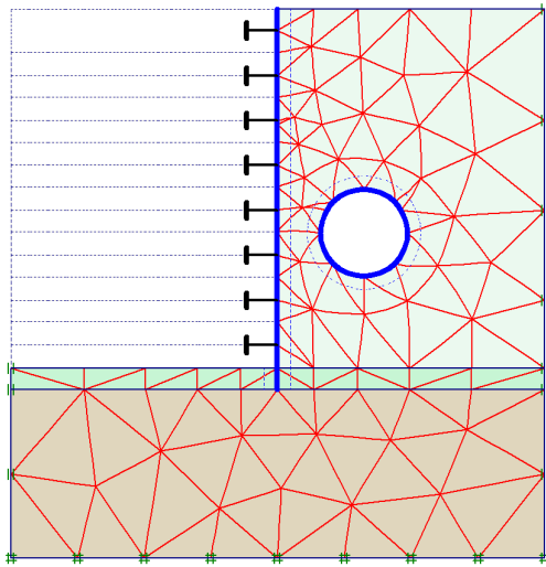
그림 4. 유한요소 해석망 및 경계조건
