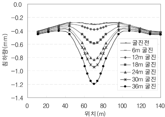
그림 14. 지하철 2호선 상부의 지표침하
