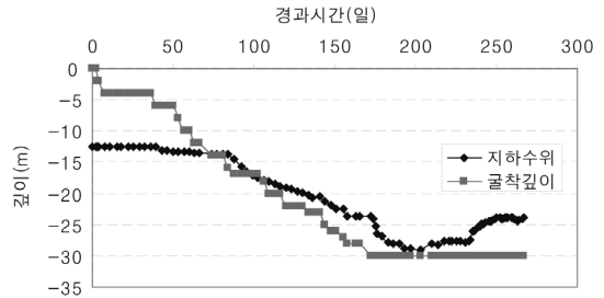
그림 2. TRcM 구간 계측자료 1
