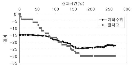
그림 3. TRcM 구간 계측자료 2
