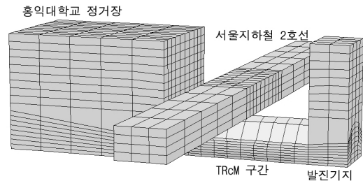
그림 5. 해석모델
