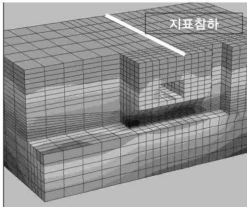
그림 11. 지표침하 측정위치
