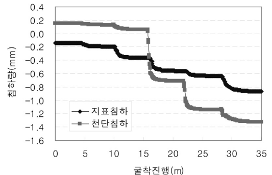
그림 10. 지하철 2호선과 공항철도 교차부의 지표침하 및 TRcM 구간 천단 침하
