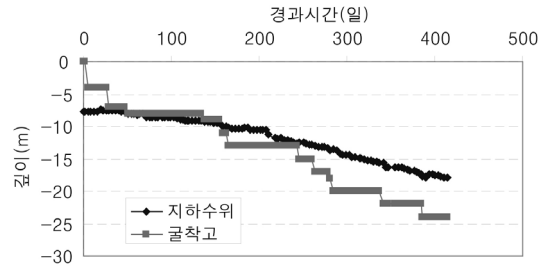
그림 1. 정거장 구간 계측자료
