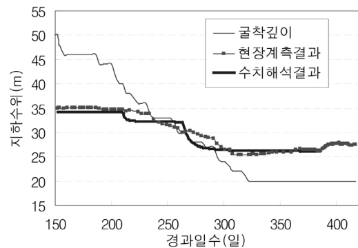
그림 6. 수치해석과 계측결과 비교
