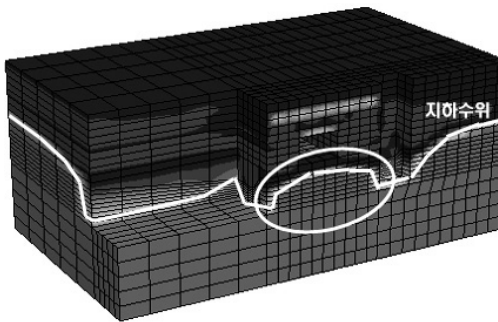
그림 7. TRcM 구간 굴착전 지하수위
