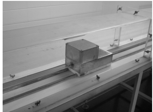
그림 6. 실험차량 전경
