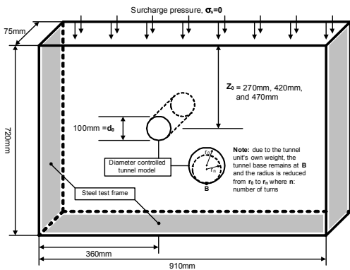
그림 4. 2차원 터널모형실험 모식도
