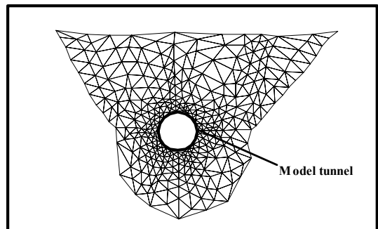
(b) 삼각형 유한요소망
