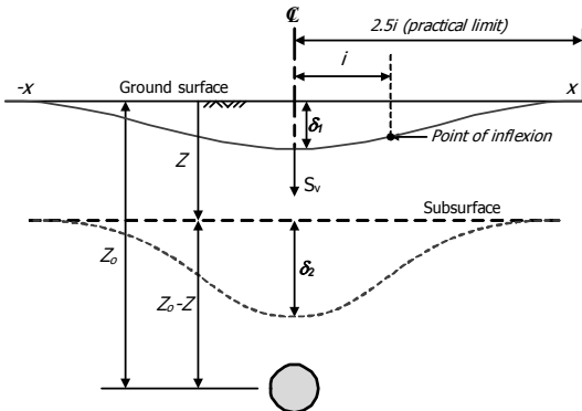
그림 2. 이론적 지표침하 및 지중침하 양상
