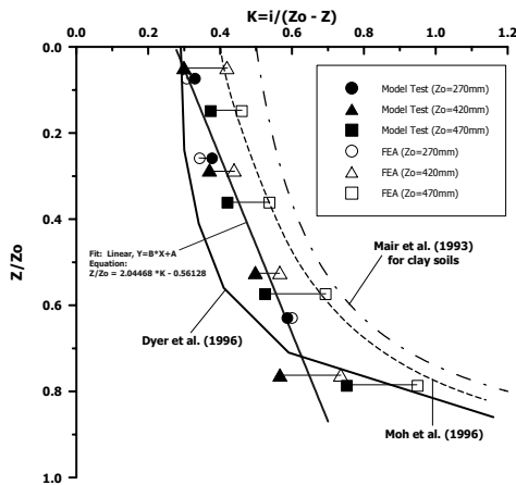
그림 12. 수치해석과 모형실험 K-Z/Z 0 관계 비교( V_L=5.83\% )
