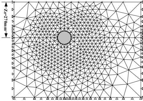
그림 7. Z_0=270 mm모형터널실험에 대한 수치해석 유한요소망
