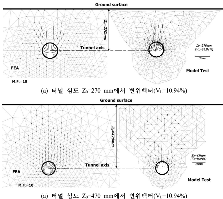
그림 8. 수치해석과 모형실험 결과 변위벡터의 비교
