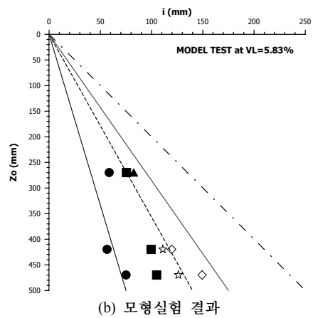
그림 11. 수치해석과 모형실험 i - Z_0 관계 비교( V_L=5.83\% )
