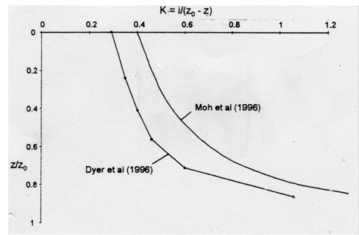
그림 3. 사질토 지반에서의 K값의 분포
