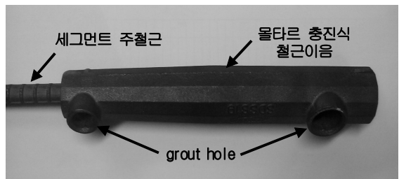
그림 4. 몰타르 충전식 철근이음
