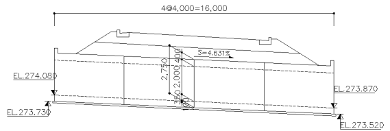
(b) 종단면도
