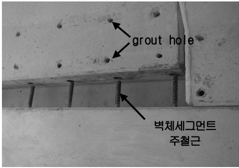
그림 5. 몰타르 충전식 철근이음 체결 전경
