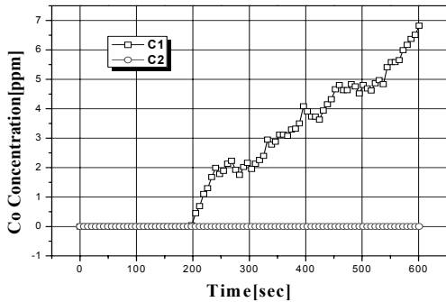
그림 3. C1 및 C2 지점에서의 시간경과별 농도변화(연직갱 A)
