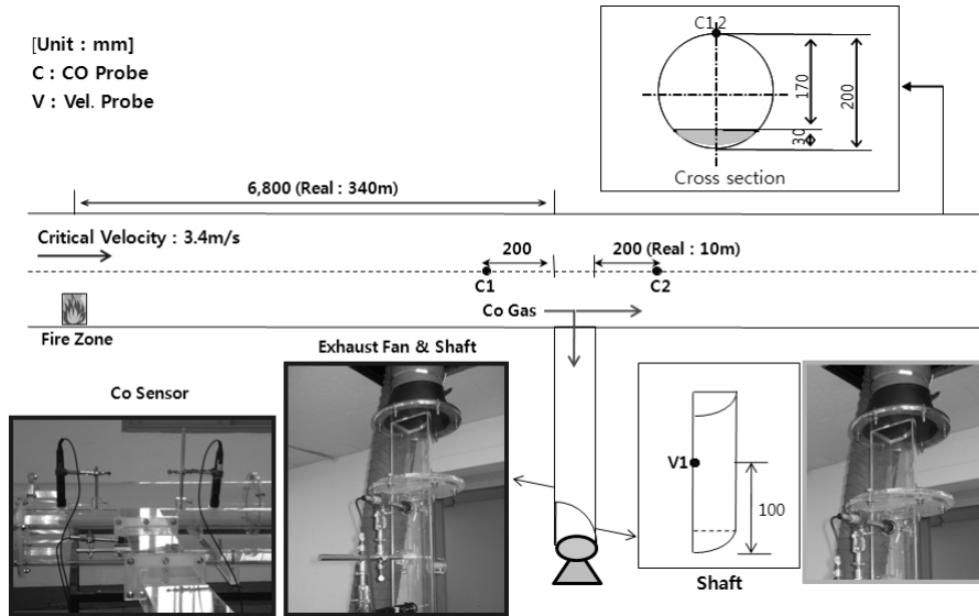
그림 5. 연직갱 배연모형 실험 모식도(연직갱 B)
