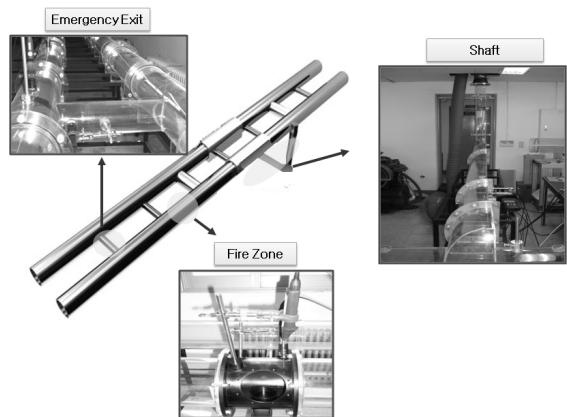
그림 1. 축소모형 실험장치
