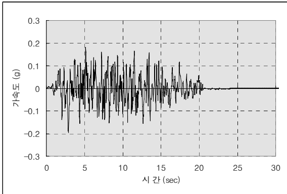
(a) 지층내 암반에서의 시간가속도 이력
