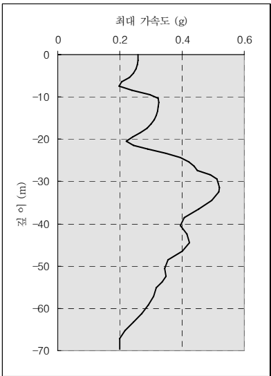
(a) 깊이별 최대가속도
