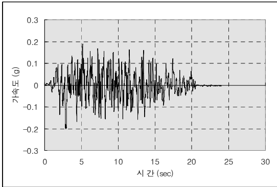
(a) 암반 노두에서의 시간가속도 이력
