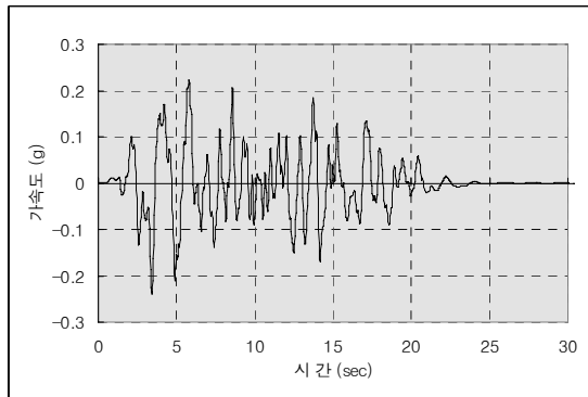
(c) 지표면에서의 시간가속도 이력
