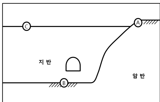
그림 11. 부지 개념도내 입력지진 통제점 위치
