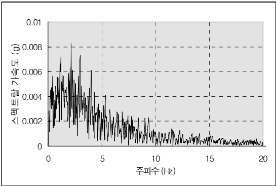
(a) 암반 노두에서의 주파수 성분
