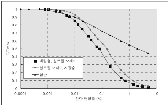
(a) 전단변형률 - G/Gmax 관계 (Idriss 등, 1992)
