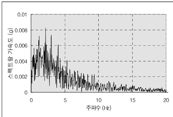
(a) 지층내 암반에서의 주파수 성분
