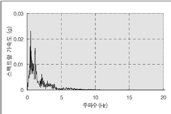
(c) 지표면에서의 주파수 성분
