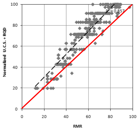
(a) 정규화한 U.C.S. + RQD
