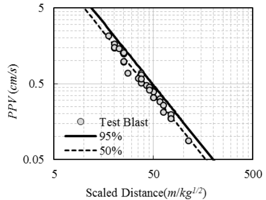
Fig. 2. Test blast result
