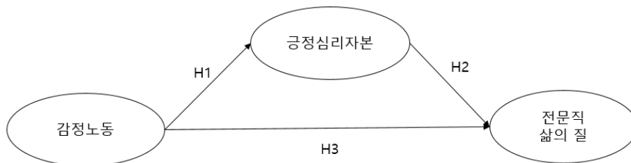
<그림 1> 연구모형
