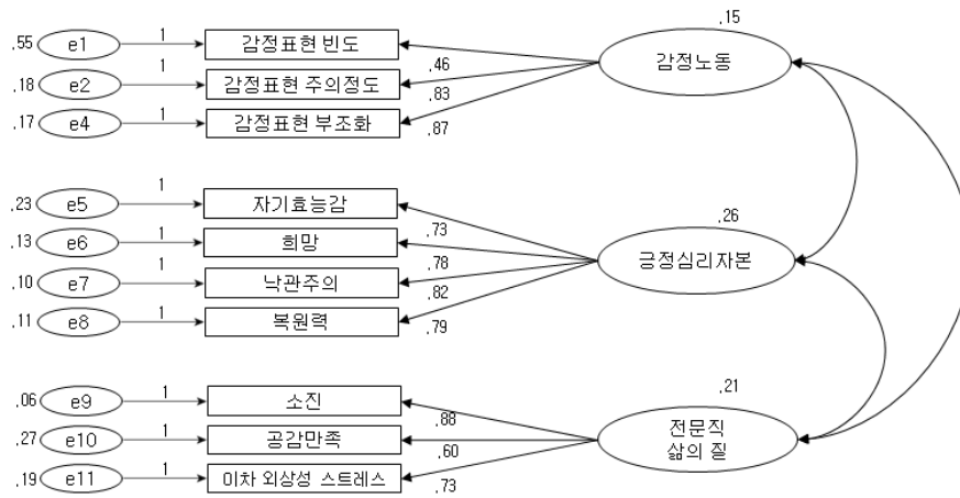
〈그림 2〉 측정모형
