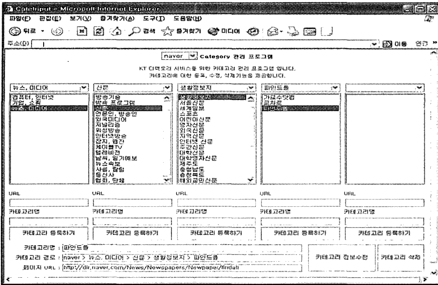
〈그림 4〉 분류항목 관리화면 설계
