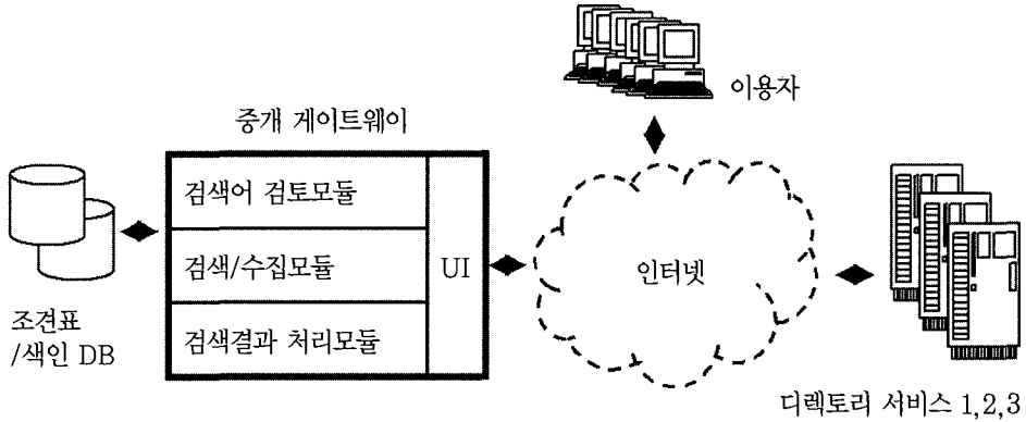
〈그림 1〉 중개 게이트웨이 서비스 모형
