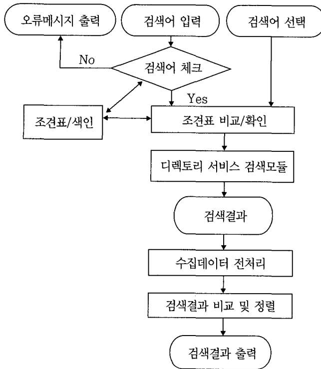
〈그림 2〉 데이터처리 흐름도
