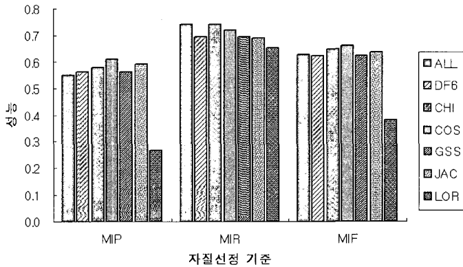
〈그림 1〉 자질선정 기준에 따른 성능
