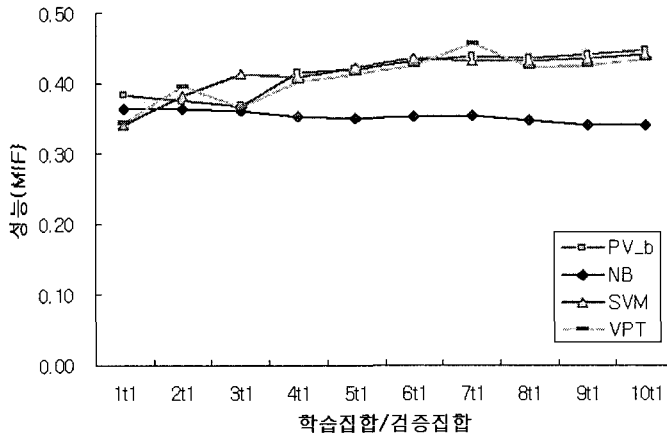
〈그림 6〉 학습집합의 변화에 따른 성능 : 프로파일 기본형(PV_b)과 다른 3개 학습기반 방법 간의 비교(마이크로 평균 F_1 )
