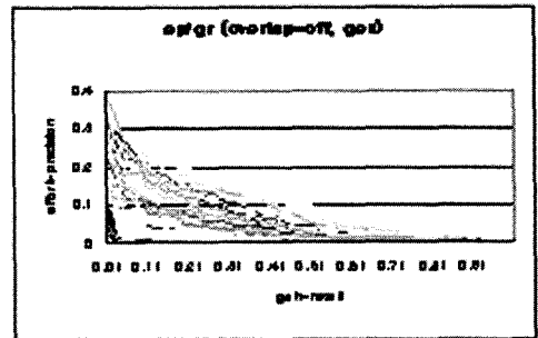
〈그림 16〉 INEX 2005에서 COS.Through의 상대적인 성능 비교: ep/gr(gen)
