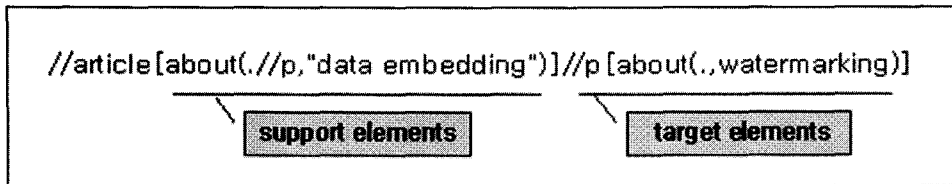
〈그림 6〉 지원 엘리먼트와 표적 엘리먼트로 구성된 질의 예
