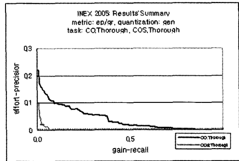
〈그림 12〉 성능비교: ep/gr(gen)
