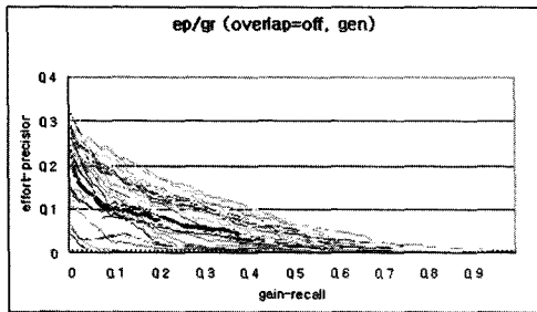
〈그림 14〉 INEX 2005에서 CO.Through의 상대적인 성능 비교: ep/gr(gen)
