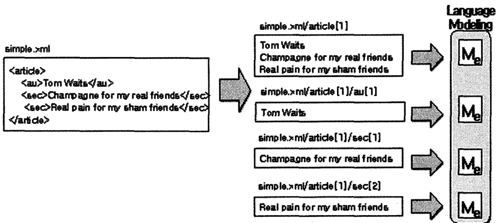
<그림 4> 구조화된 문헌의 언어모델링 단위
