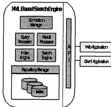
〈그림 2〉 시스템 구조
