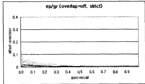
〈그림 15〉 INEX 2005에서 COS.Through의 상대적인 성능 비교: ep/gr(stict)
