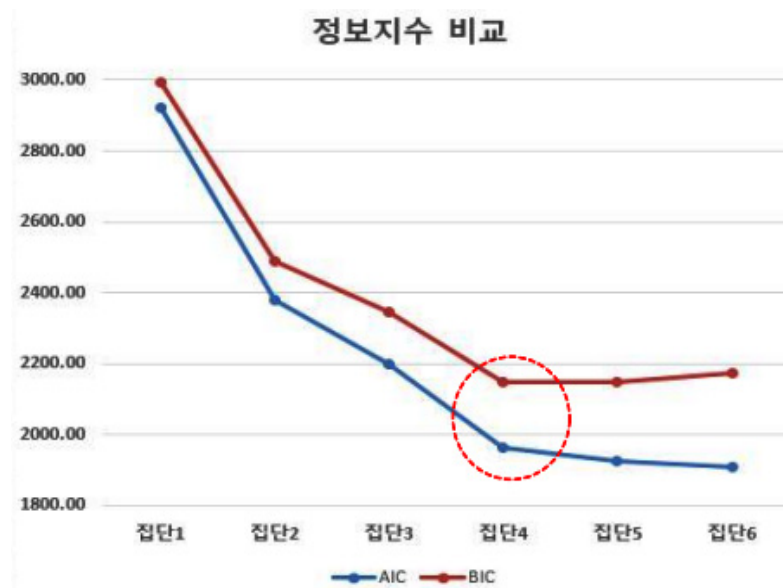
〈그림 2〉 AIC, BIC 정보지수 비교
