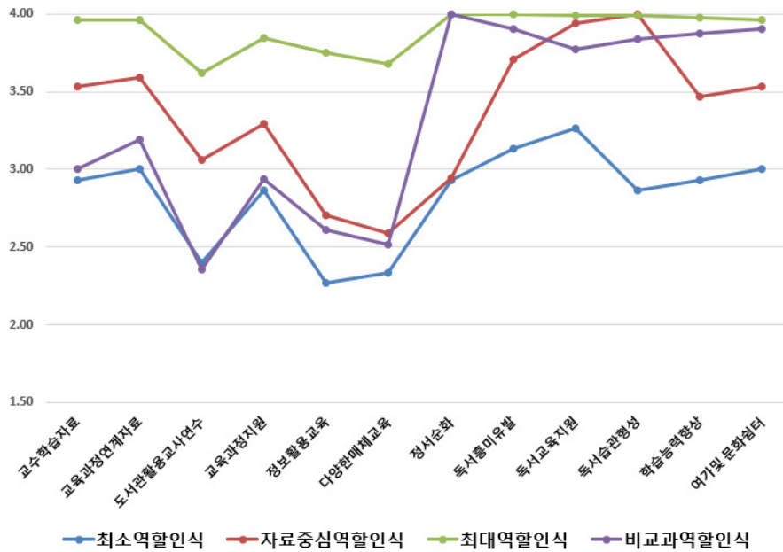
〈그림 3〉 학교도서관 역할 인식에 따른 유형 분류 그래프 모형
