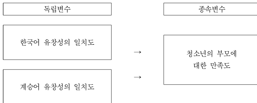
그림 1. 연구모형
