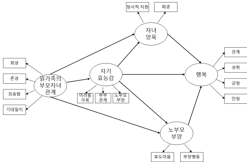
그림 1. 연구모형
