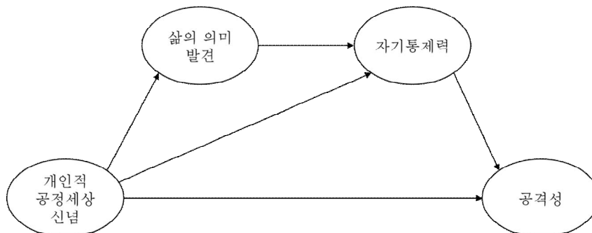
그림 1. 연구모형
