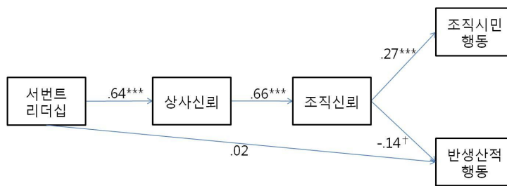
그림 5. 부분매개모형 3
