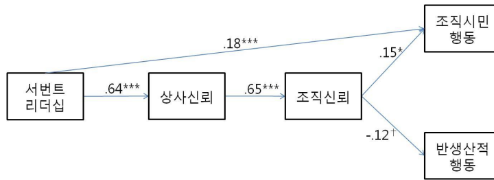
그림 4. 부분매개모형 2
