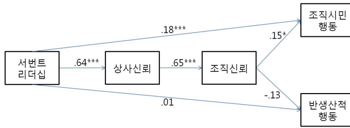
그림 3. 부분매개모형 1
