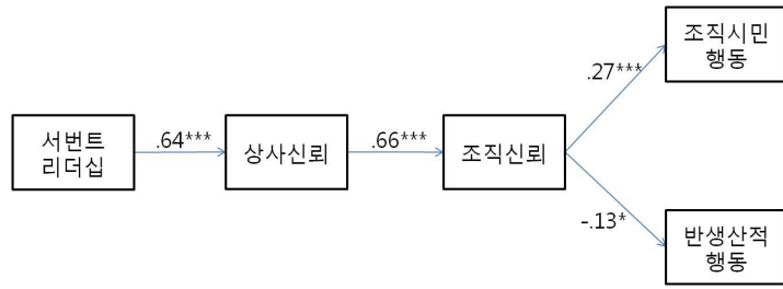
그림 2. 완전매개모형
